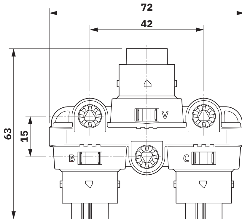
Maßzeichnung
