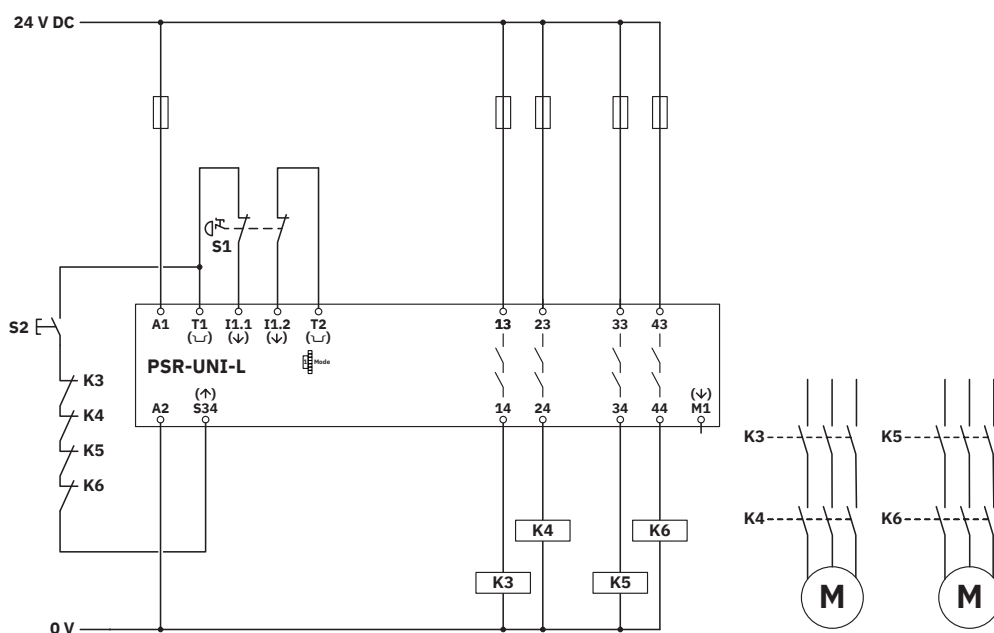
Schaltplan
