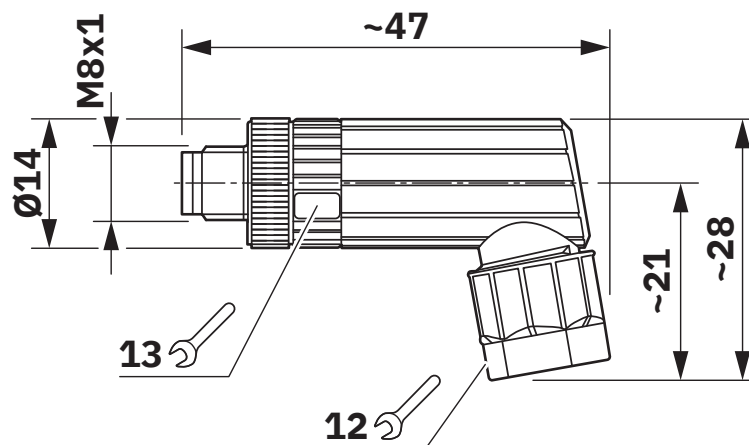
Maßzeichnung
