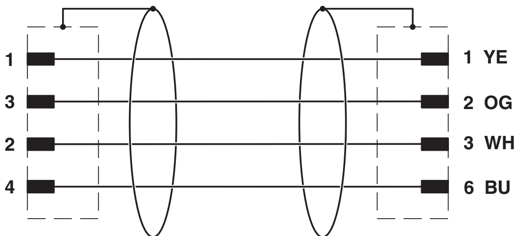
Kontaktbelegung des M8- und RJ45-Steckers
