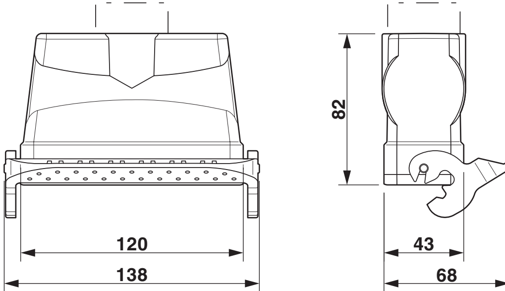
Maßzeichnung
