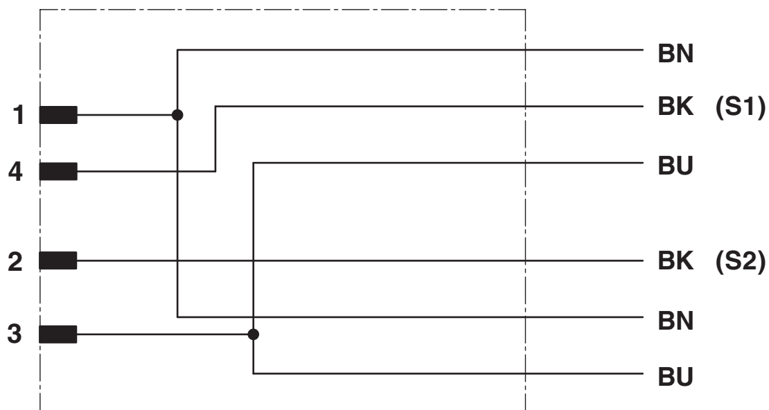
Kontaktbelegung des M8 Y-Verteilers
