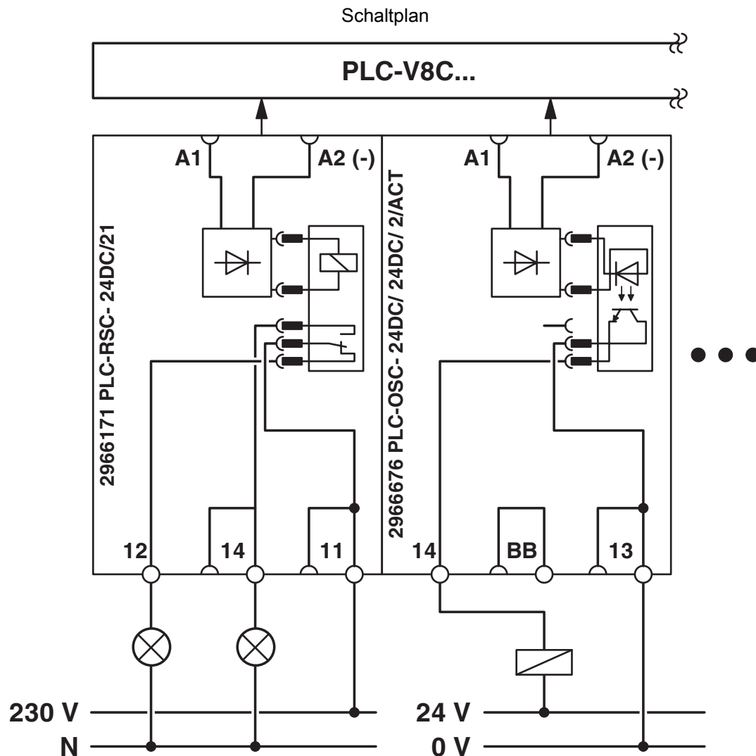
Prinzipschaltplan: Ausgänge über PLC-INTERFACE am Beispiel einer Ausgabeklemme mit Relais, 1 Wechsler und einer Ausgabeklemme mit Solid-State Relais.
