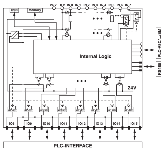
Schaltplan
