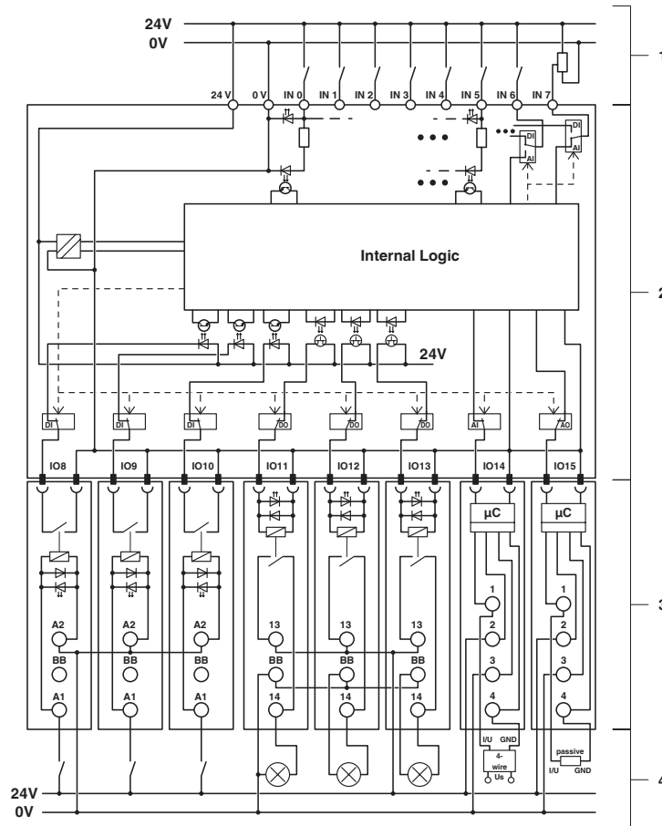
Schaltplan
