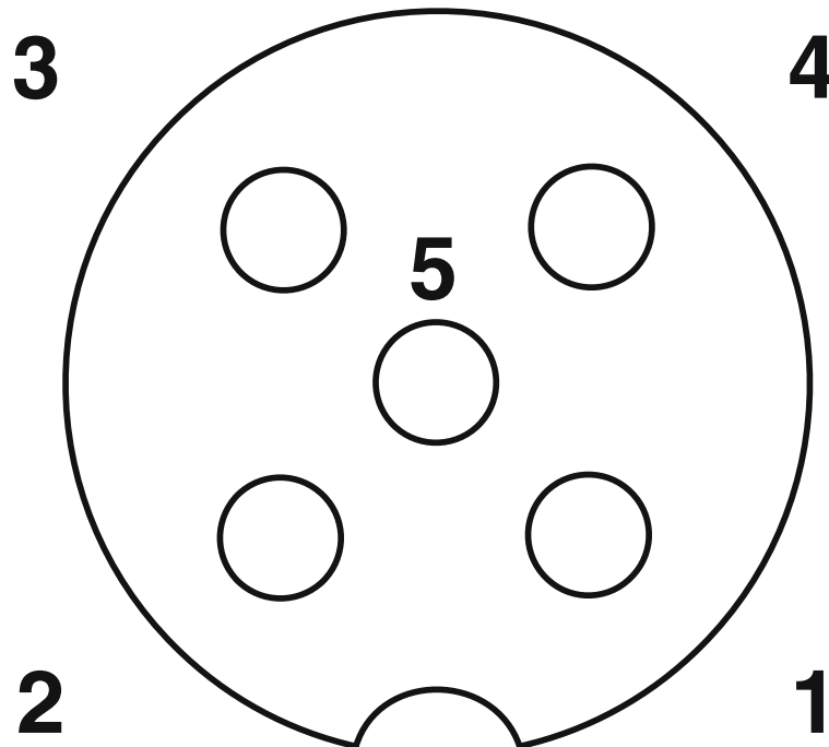
Schemazeichnung
