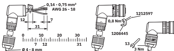
Funktionszeichnung
