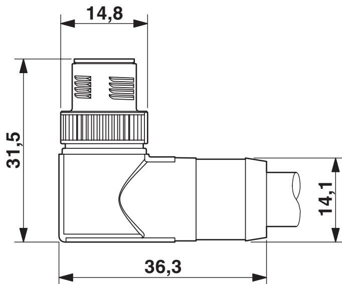
Maßzeichnung
