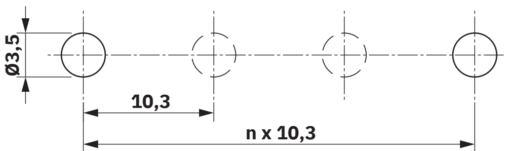
Maßzeichnung
