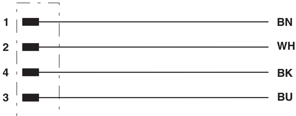
Schaltplan
