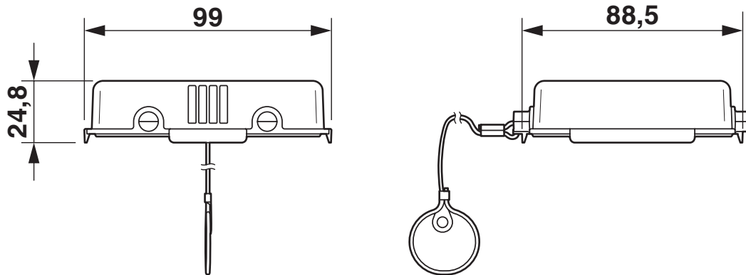
Maßzeichnung
