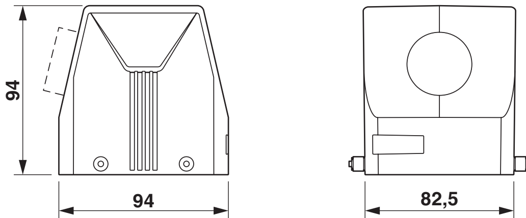
Maßzeichnung
