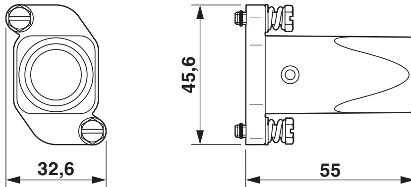
Maßzeichnung
