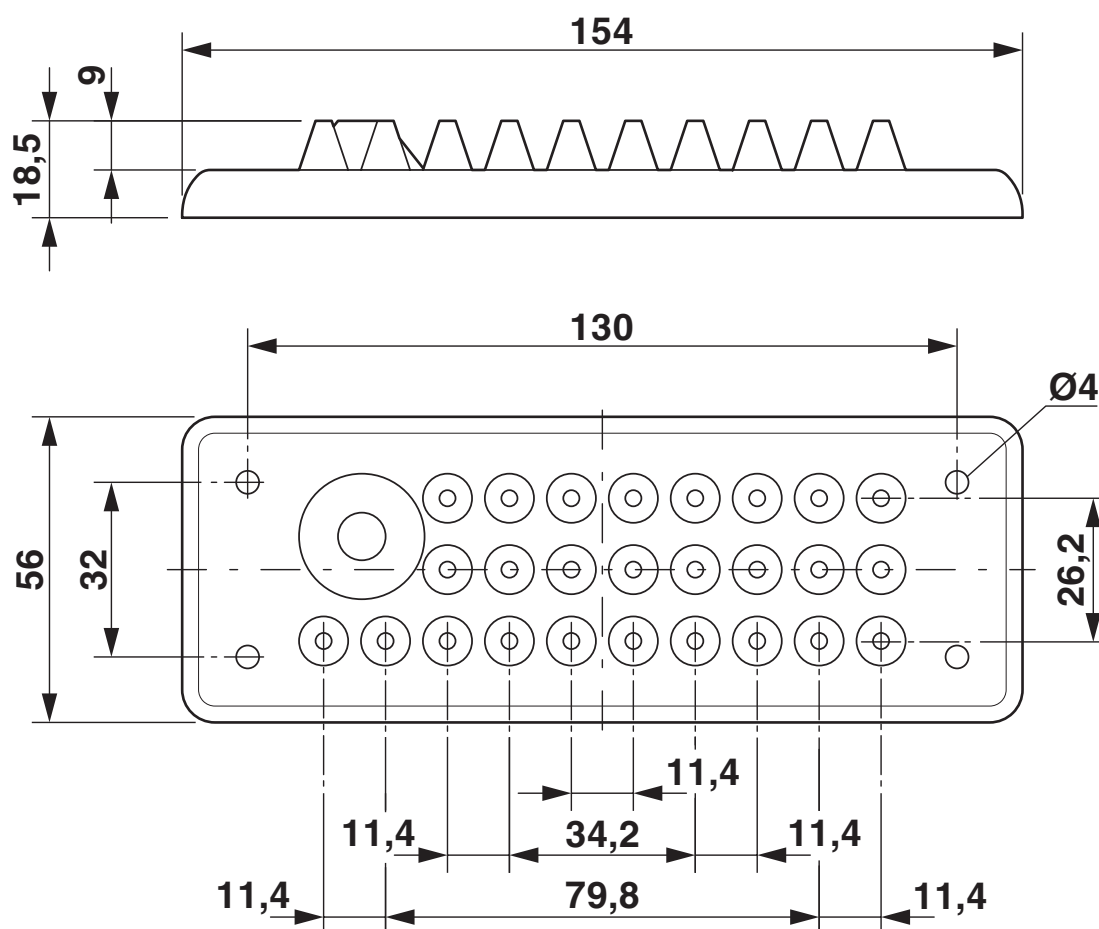
Maßzeichnung
