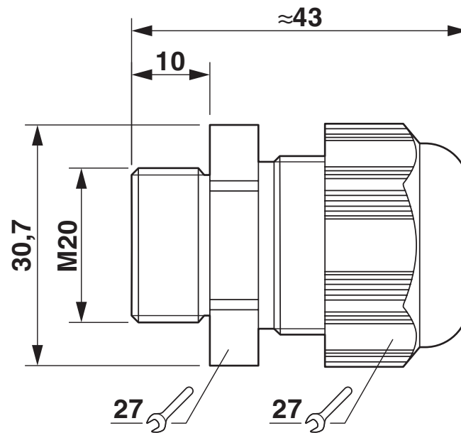
Maßzeichnung
