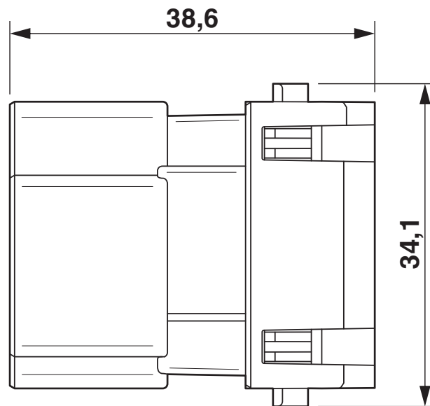
Maßzeichnung
