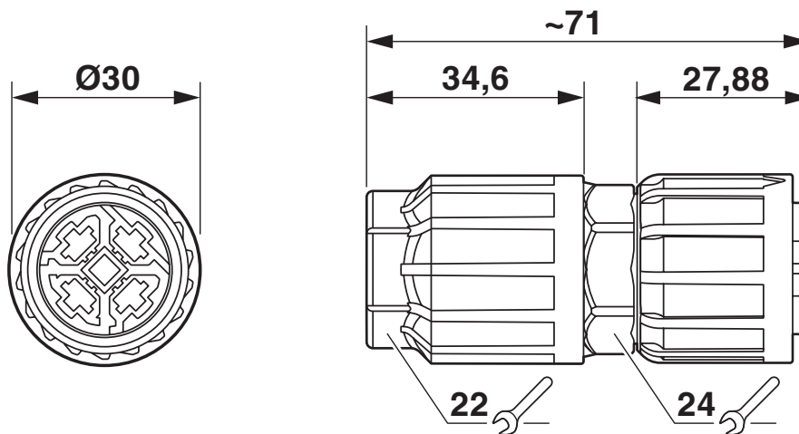
Maßzeichnung
