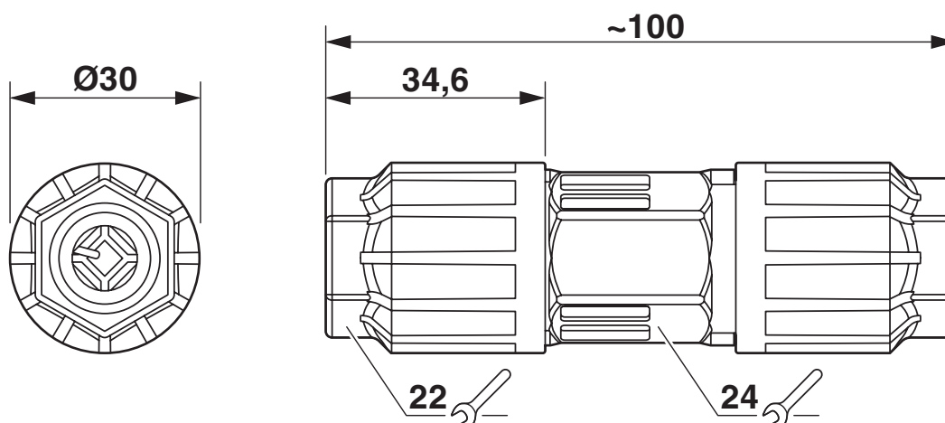
Maßzeichnung
