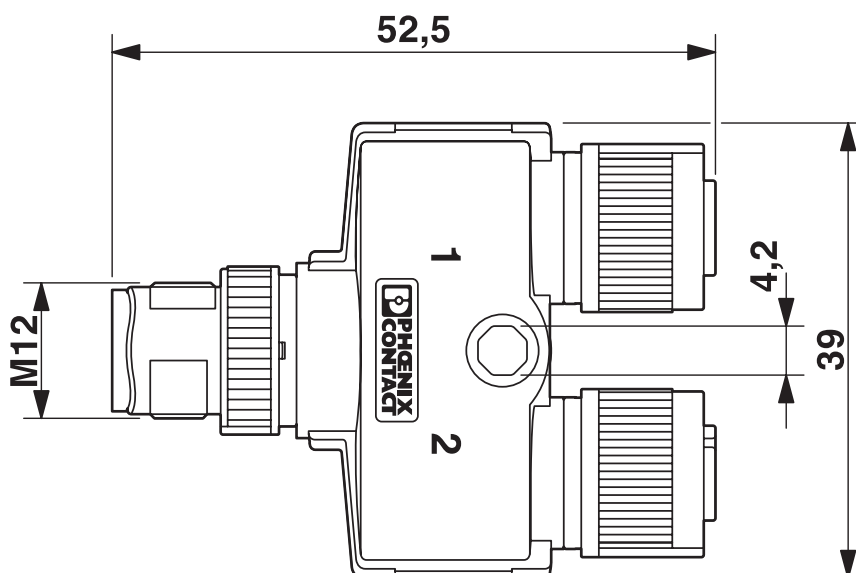
Maßzeichnung
