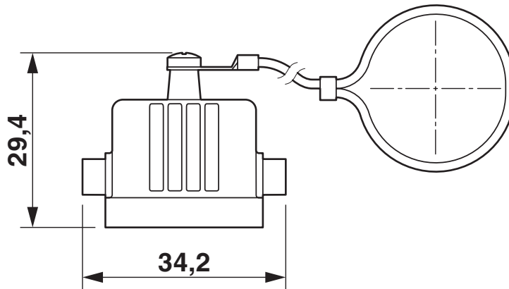
Maßzeichnung
