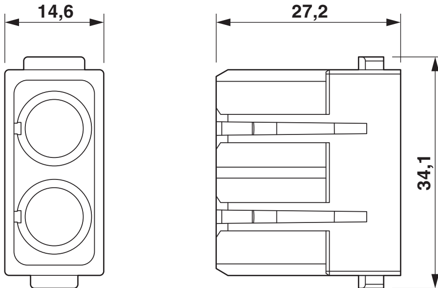
Maßzeichnung
