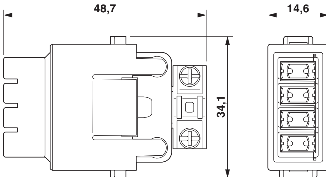
Maßzeichnung
