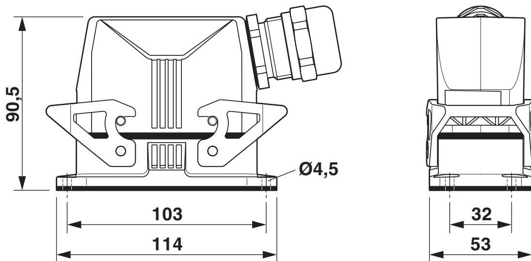
Maßzeichnung
