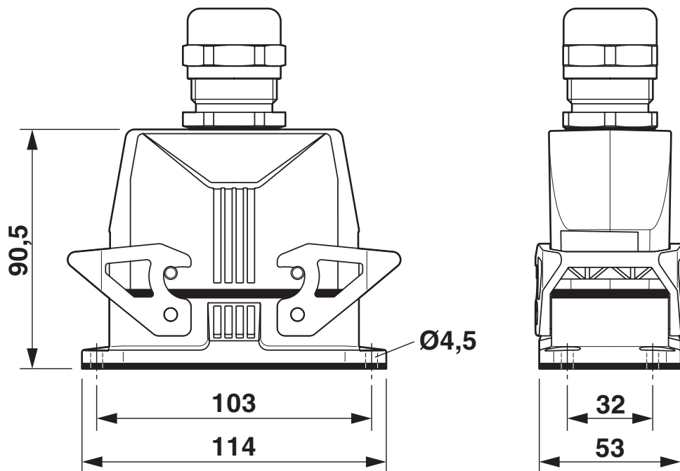
Maßzeichnung
