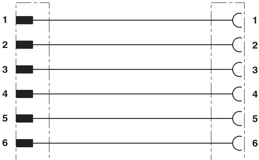
Schaltplan
