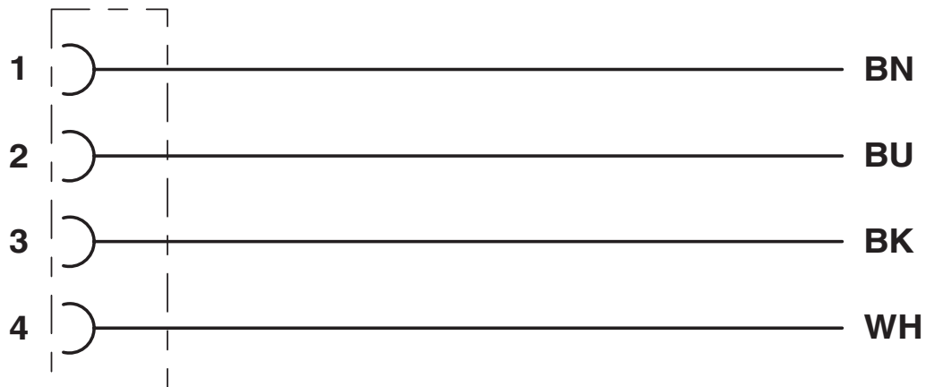
Schaltplan
