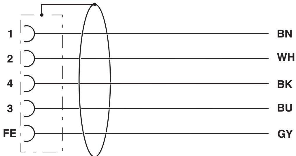
Schaltplan
