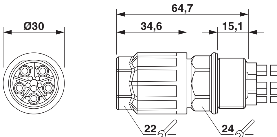
Maßzeichnung
