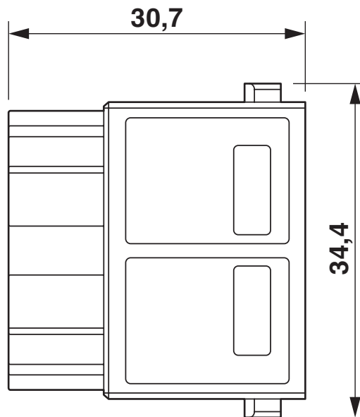
Maßzeichnung
