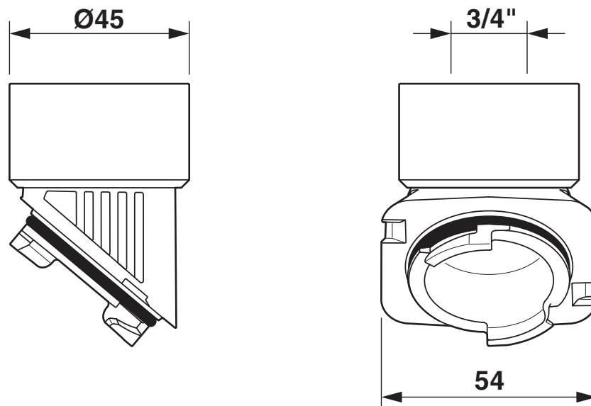
Maßzeichnung
