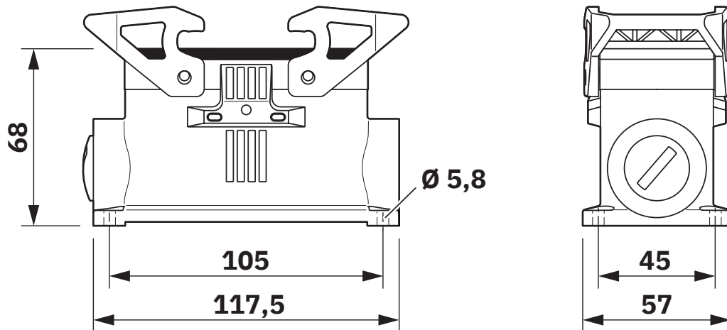
Maßzeichnung
