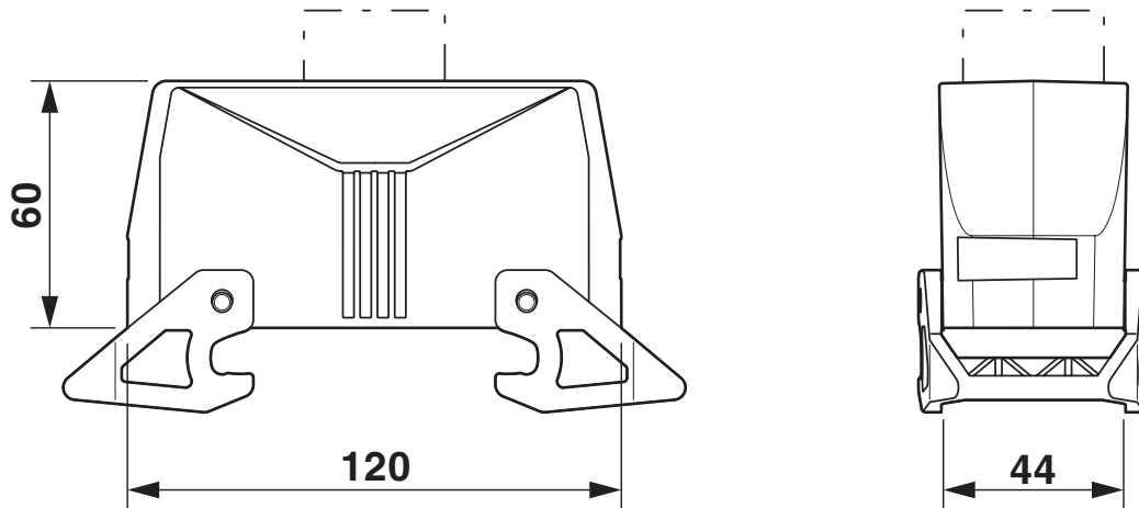
Maßzeichnung
