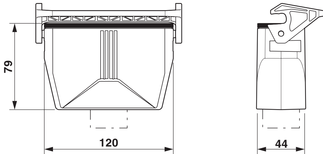
Maßzeichnung
