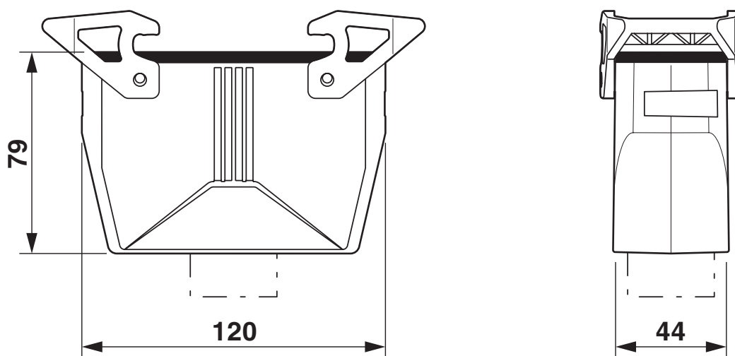
Maßzeichnung
