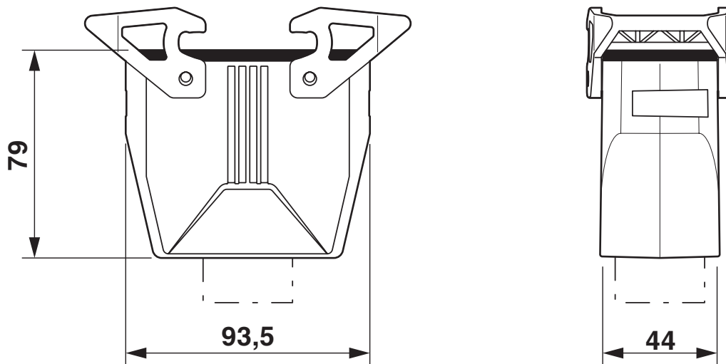
Maßzeichnung
