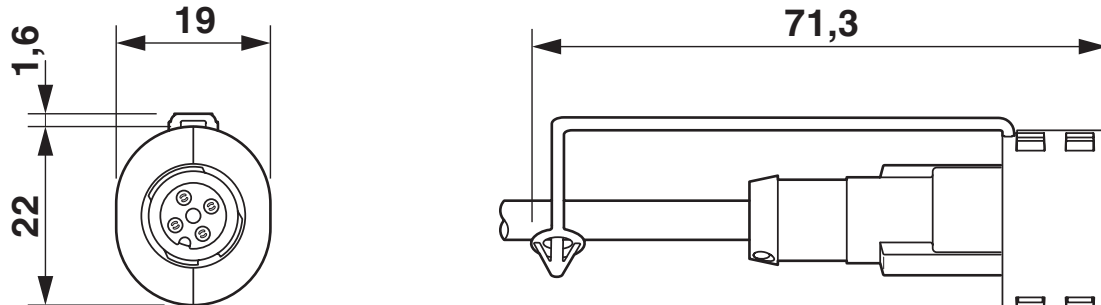
Maßzeichnung
