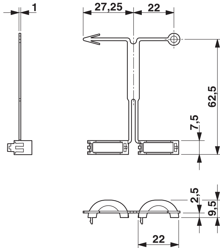
Maßzeichnung
