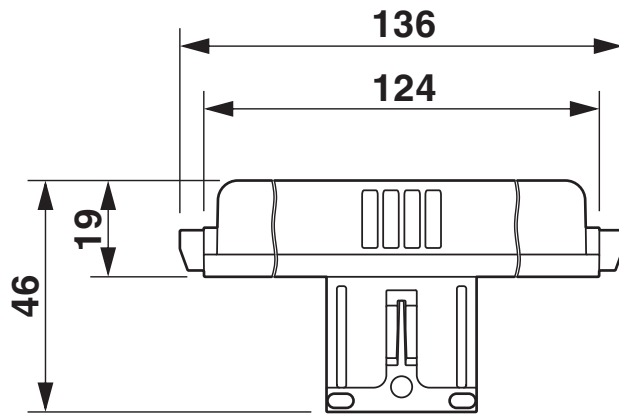
Maßzeichnung
