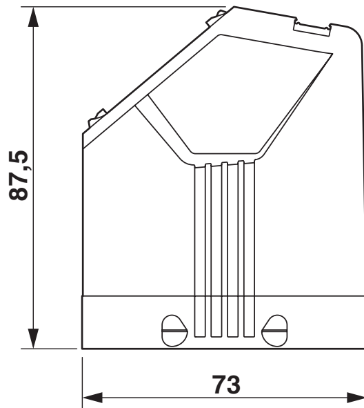
Maßzeichnung
