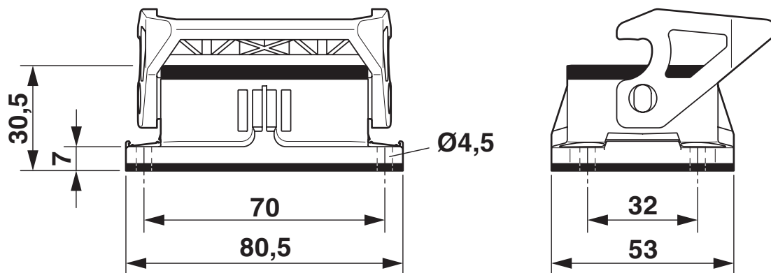
Maßzeichnung
