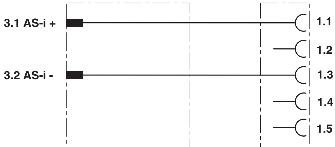
Kontaktbelegung des AS-Interface Verteilers
