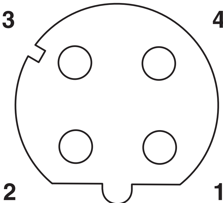
Schemazeichnung
