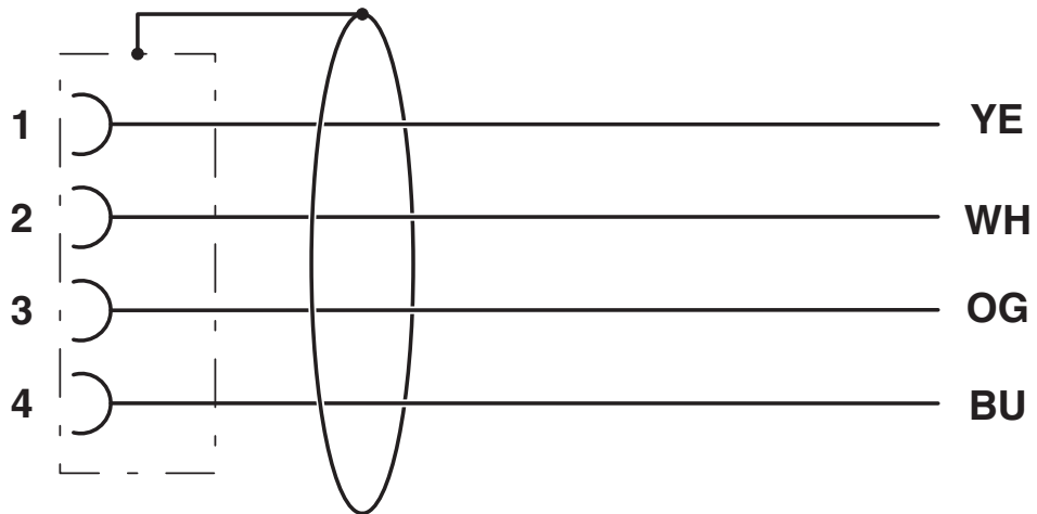
Kontaktbelegung der M12-Buchse
