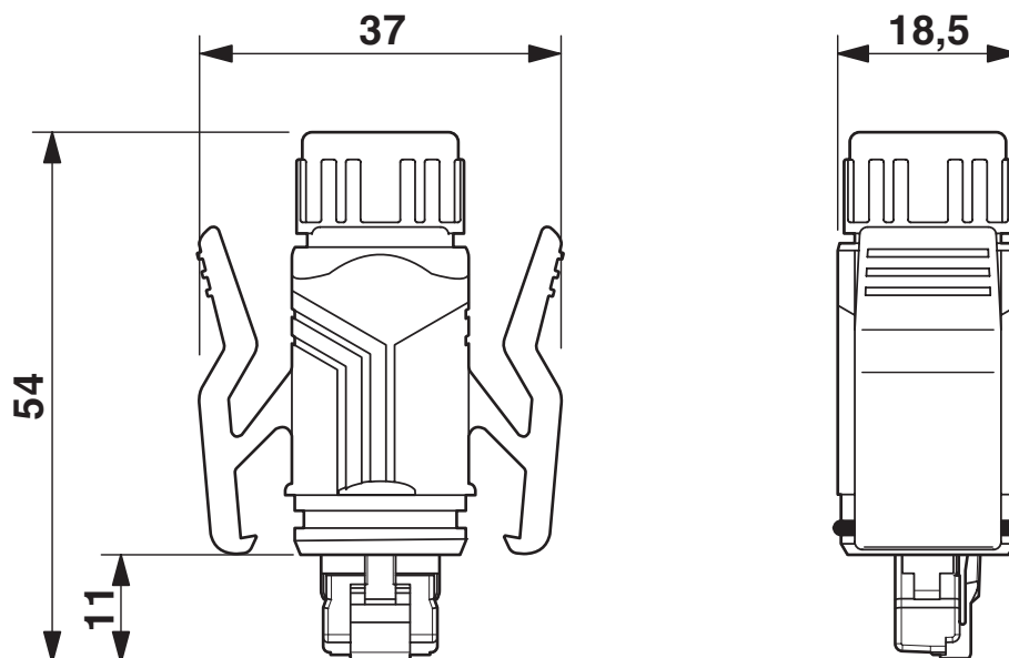
Maßzeichnung
