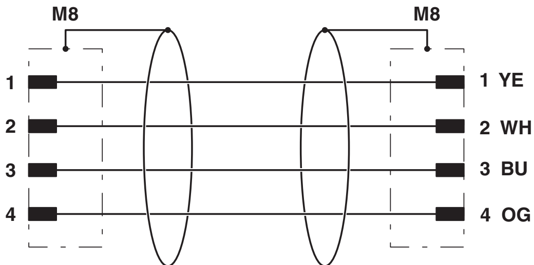
Kontaktbelegung der M8-Stecker
