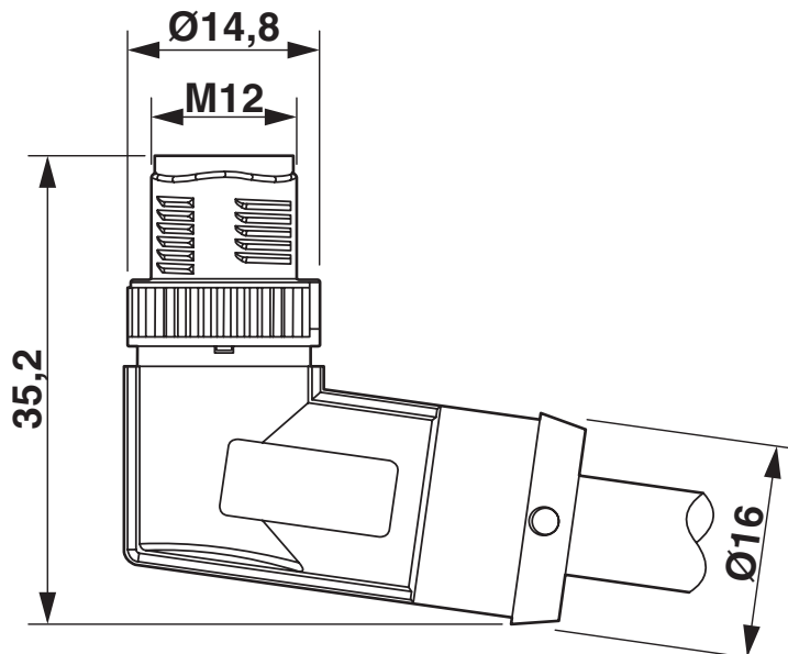
Maßzeichnung
