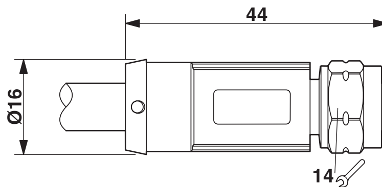
Maßzeichnung
