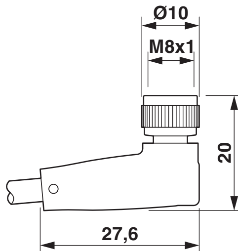
Maßzeichnung
